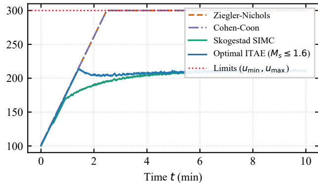
(d) Fouled Jacket (70%UA): Coolant q_j
