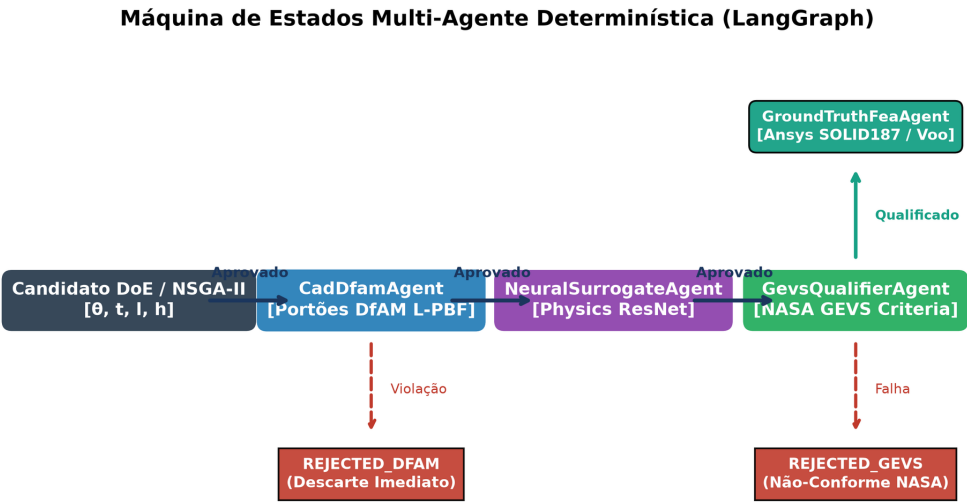
Figura 10 – Grafo acíclico determinístico de fluxo de dados (LangGraph) para triagem geométrica e qualificação aeroespacial do chassi
