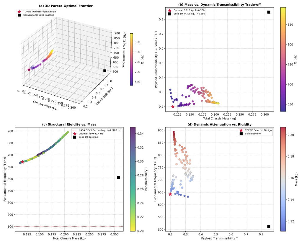
Figura 11 – Fronteira de Pareto multiobjetivo (massa estrutural \times transmissibilidade dinâmica) e correlações paramétricas obtidas pelo algoritmo NSGA-II
