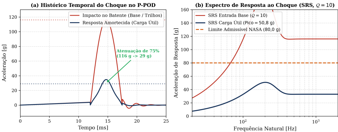
Figura 14 – Resposta dinâmica ao choque transiente de ejeção do dispensador P-POD: (a) histórico temporal da aceleração de impacto contra o batente mecânico amortecido; (b) Espectro de Resposta ao Choque (SRS, Q = 10 ) comparando a excitação de base, a resposta atenuada na carga útil e o teto normativo da NASA
