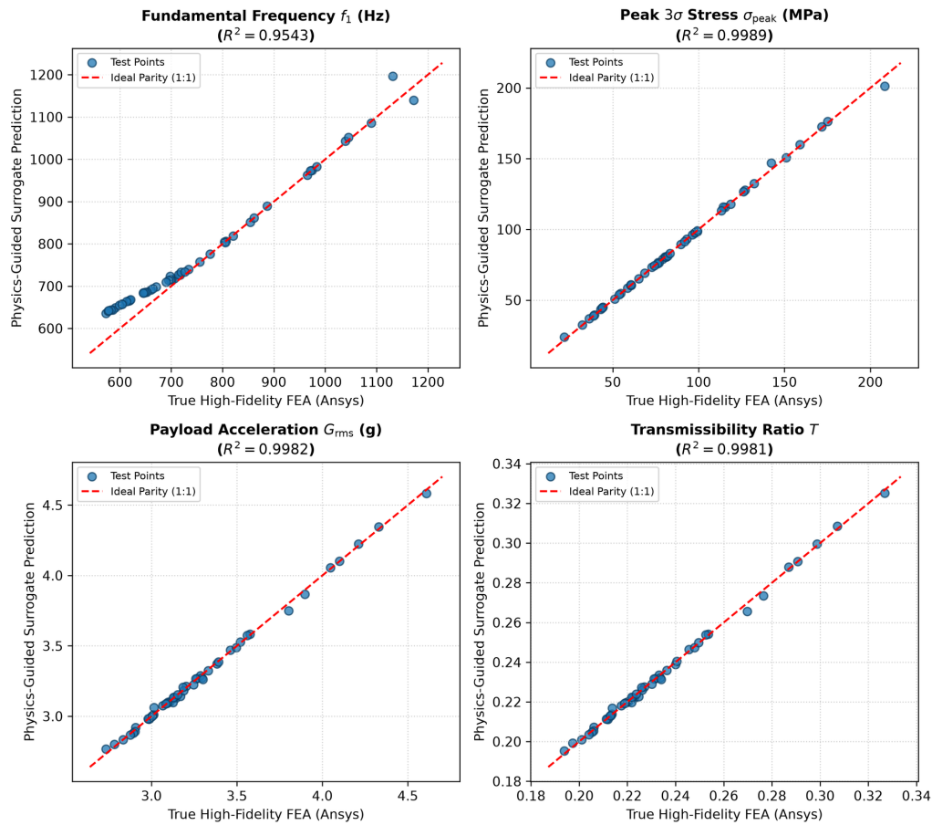
Figura 9 – Gráficos de paridade comparando previsões neurais residuais e respostas numéricas de alta ordem (Ansys MAPDL) no conjunto de teste
