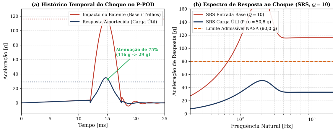
Figura 13 – Resposta dinâmica ao choque transiente de ejeção do dispensador P-POD: (a) histórico temporal da aceleração de impacto contra o batente mecânico amortecido; (b) Espectro de Resposta ao Choque (SRS, Q = 10 ) comparando a excitação de base, a resposta atenuada na carga útil e o teto normativo da NASA
