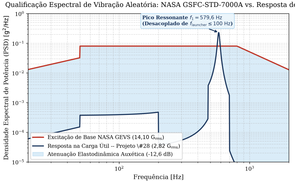
Figura 12 – Densidade Espectral de Potência (PSD) de qualificação aeroespacial: excitação estocástica de base NASA GSFC-STD-7000A (14,10 G_{rms} ) versus resposta atenuada na interface da carga útil para o Projeto #28 (2,82 G_{rms} )
