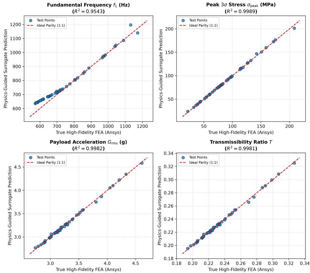
Figura 8 – Gráficos de paridade comparando previsões neurais residuais e respostas numéricas de alta ordem (Ansys MAPDL) no conjunto de teste
