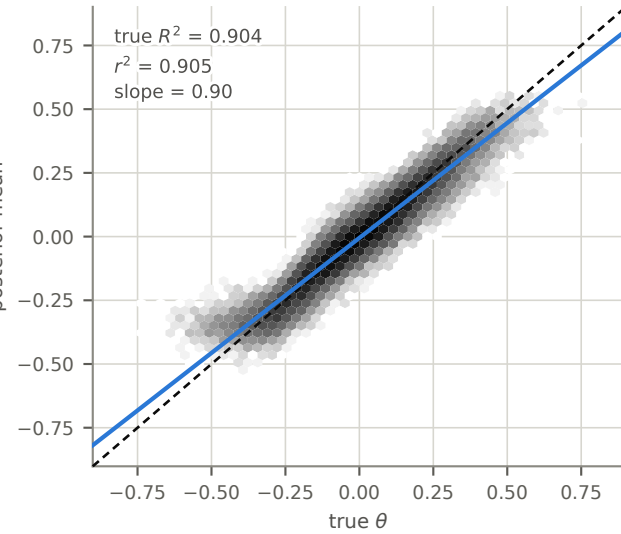
ArmToken-NPE
