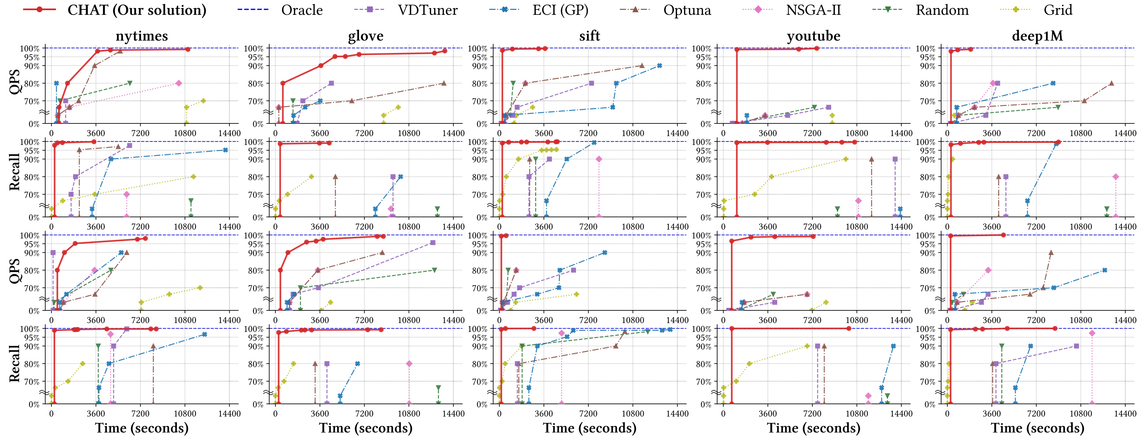
Hnswlib
