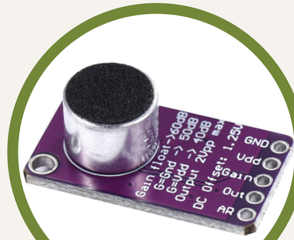
MAX9814 Micrófono
