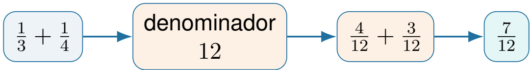
Figura 12: Esquema de combinacion de cantidades: situacion 02 de la pizza.
