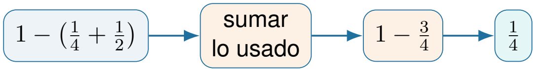
Figura 13: Esquema de complemento: situacion 03 de caramelos.
