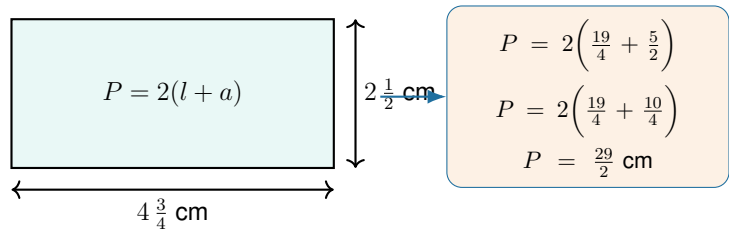
Figura 14: Situacion 10: perimetro de un rectangulo con medidas fraccionarias.
