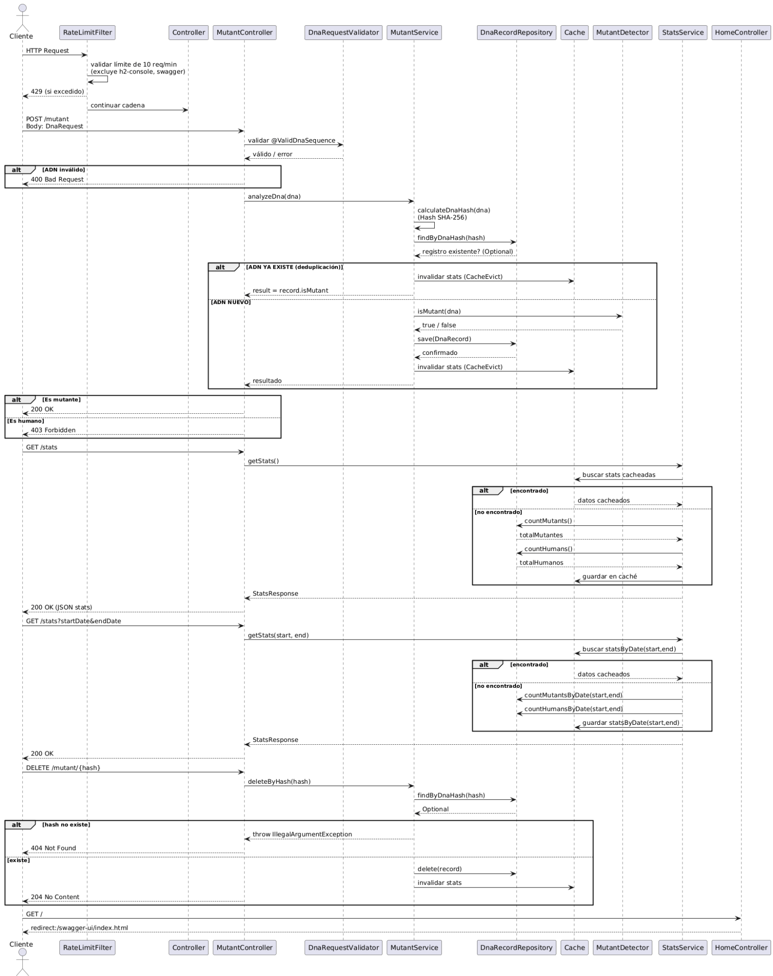
DETECTOR DE MUTANTES - Diagrama de Secuencia Completo (Versión Final)
