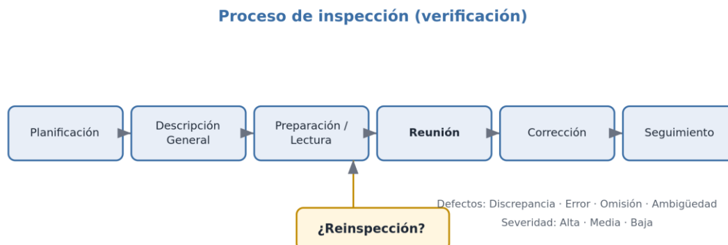
Fig. 2.6. Proceso de inspección para la verificación de los modelos, con sus etapas y la clasificación de defectos por tipo y severidad.
