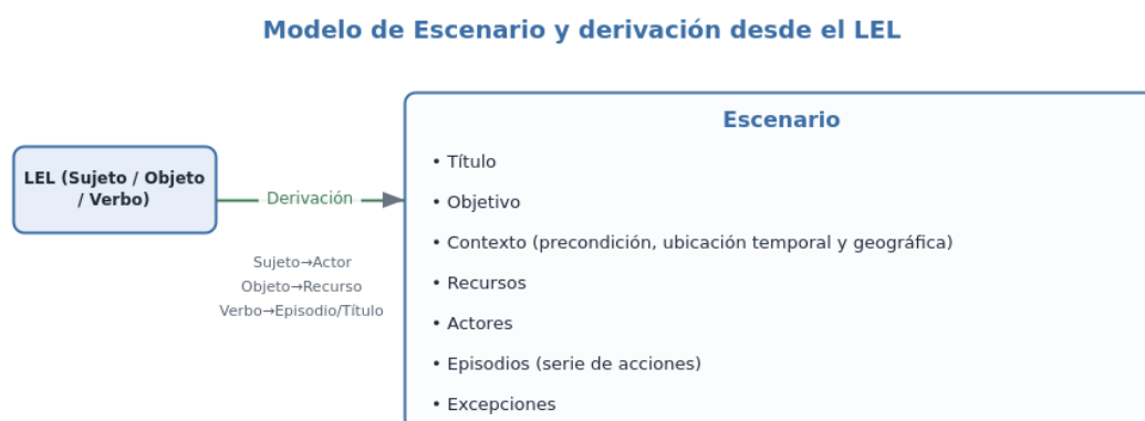
Fig. 2.5. Componentes del modelo de Escenario y su derivación desde el LEL: los símbolos de tipo Sujeto tienden a convertirse en actores, los de tipo Objeto en recursos, y los de tipo Verbo en episodios o títulos de escenario.
