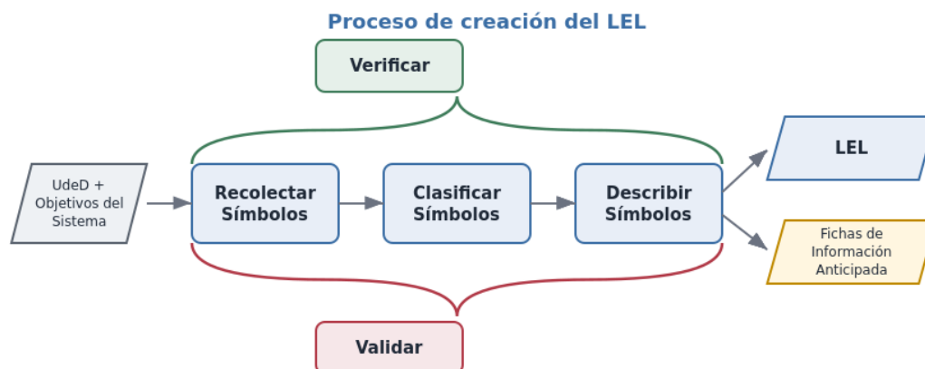
Flujo principal (Recolectar→Clasificar→Describir) con retroalimentación por verificación y validación.
