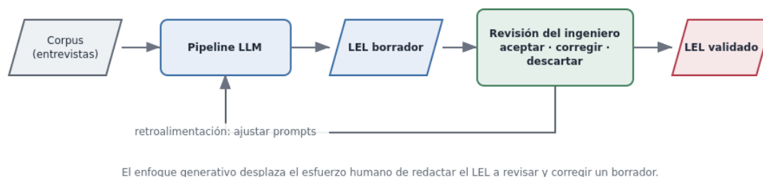
Fig. 8.1. El LEL generado y la revisión humana: el enfoque generativo desplaza el esfuerzo del ingeniero de redactar el LEL desde cero a revisar y corregir un borrador.
