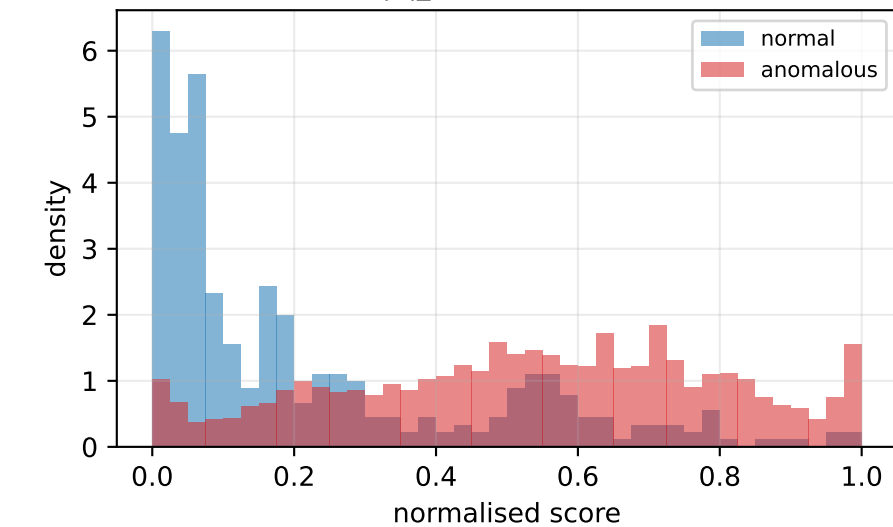
|S|_1 (AUC=0.812)
