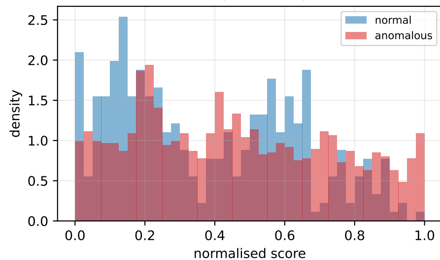
LS (AUC=0.418)
