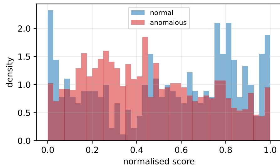
|S|_1 (AUC=0.812)
