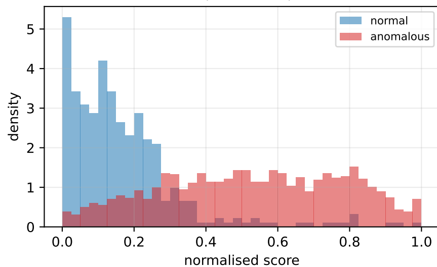
raw_to_S (AUC=0.546)
