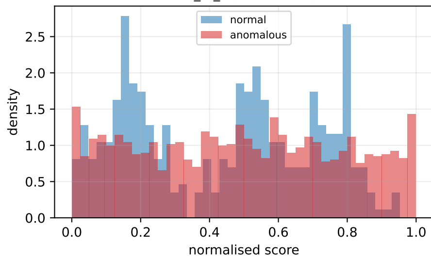
raw_to_S (AUC=0.546)
