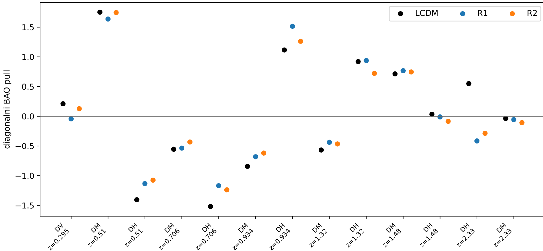
DESI DR2 BAO rezidua
