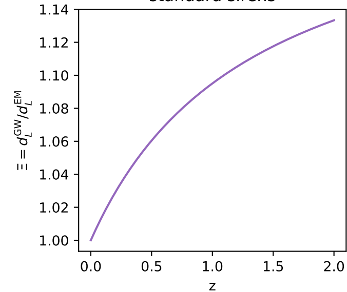
standard sirens
