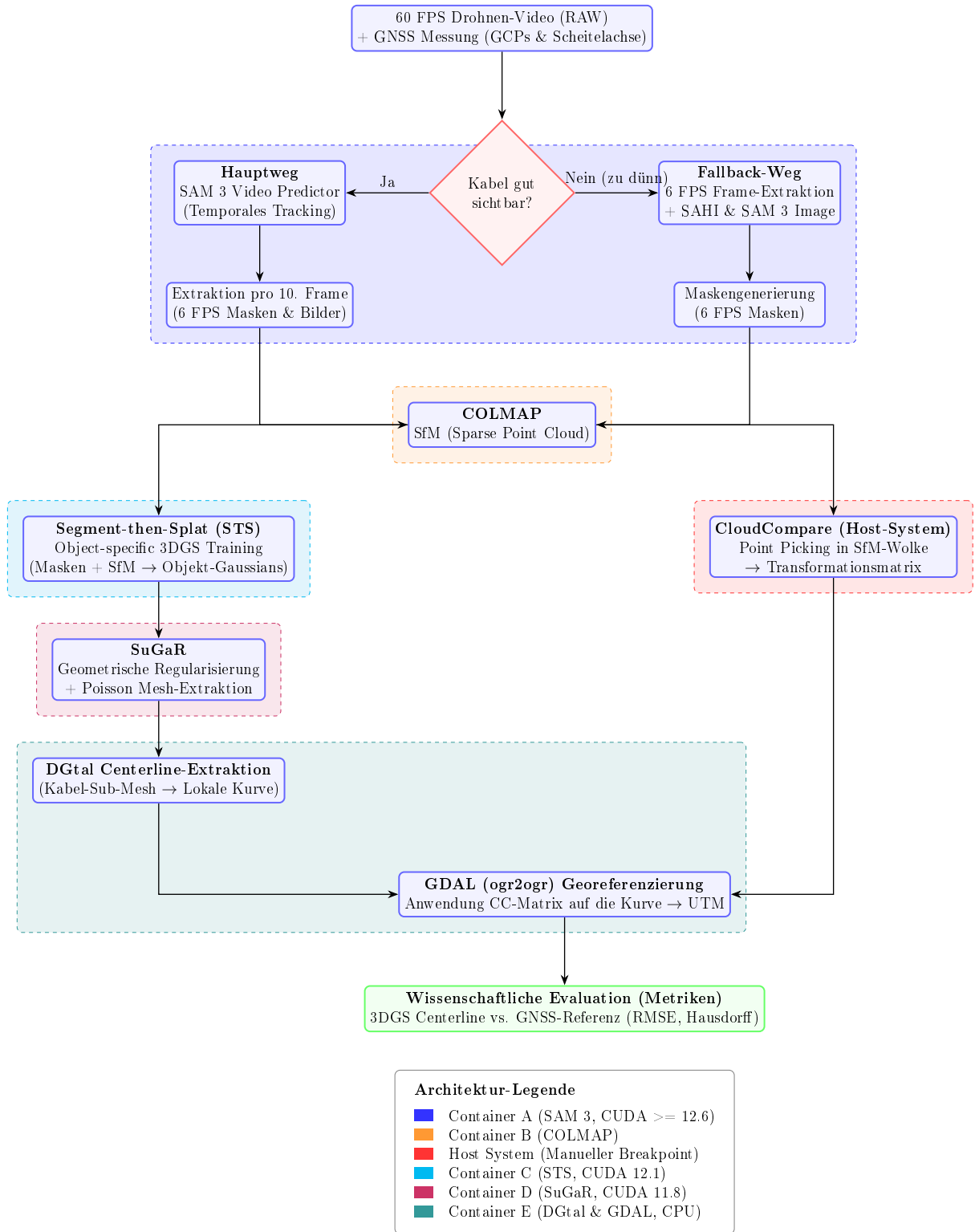
Figure 1: Microservice-Architektur (v4): 5-Container-Pipeline mit Segment-then-Splat für objektspezifisches Training und SuGaR für geometrisches Meshing.
