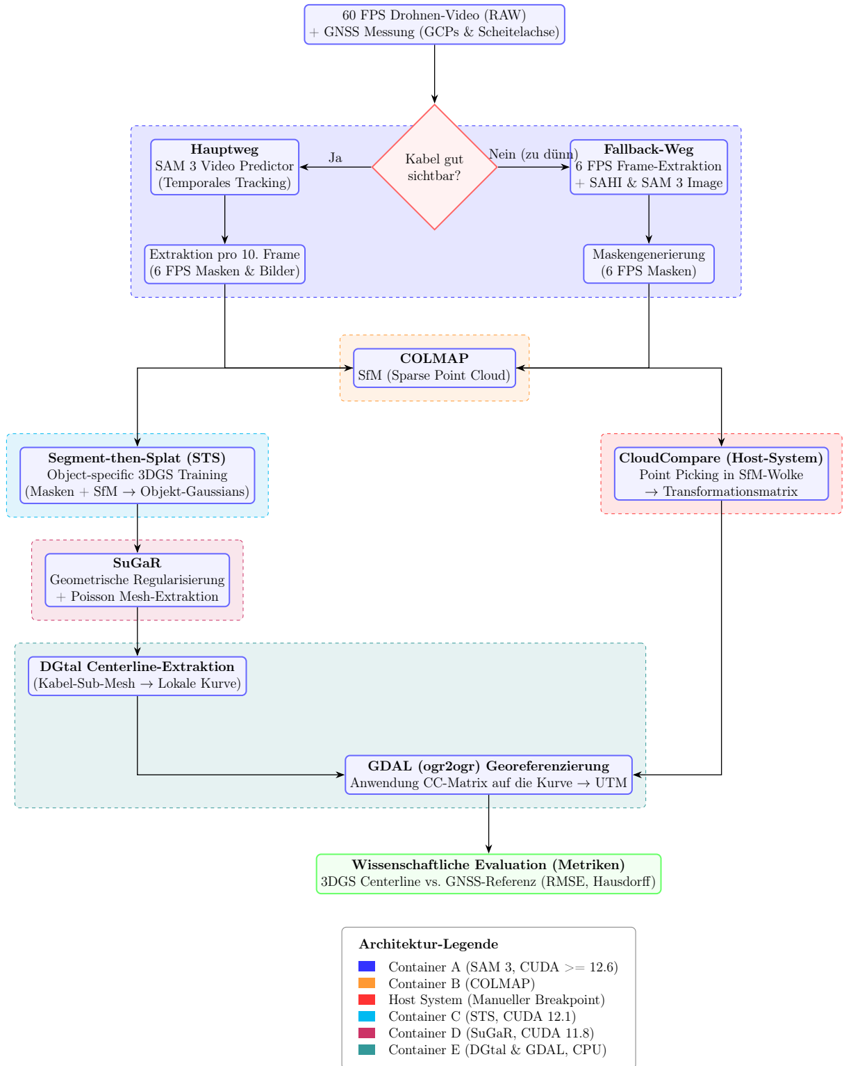
Abbildung 7: Microservice-Architektur (v4): 5-Container-Pipeline mit Segment-then-Splat für objektspezifisches Training und SuGaR für geometrisches Meshing.
