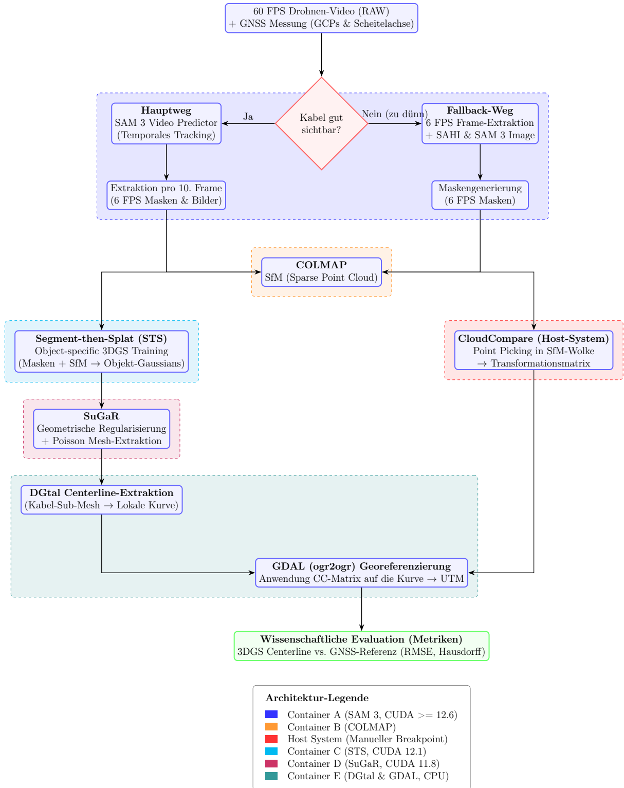
Abbildung 5: Microservice-Architektur (v4): 5-Container-Pipeline mit Segment-then-Splat für objektspezifisches Training und SuGaR für geometrisches Meshing.
