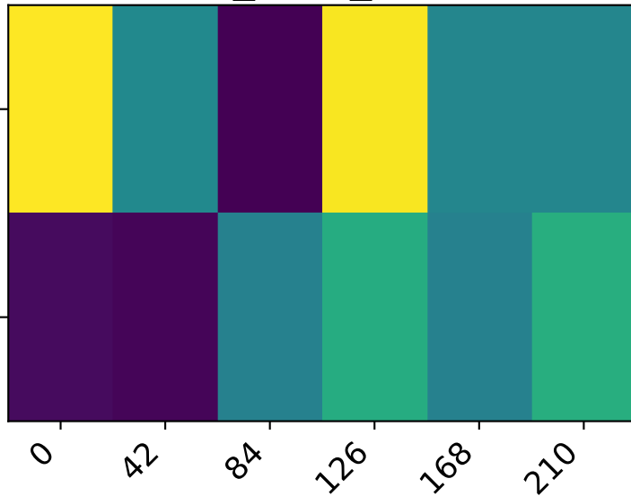
rcsums_rc14_rcrand13
