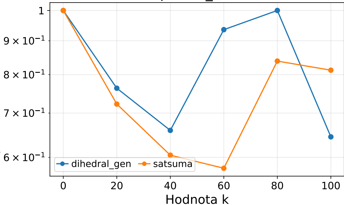
queens_n10
