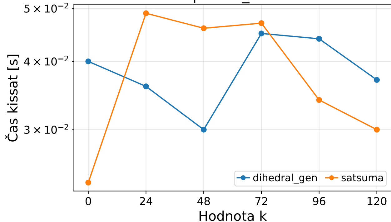
queens_n11
