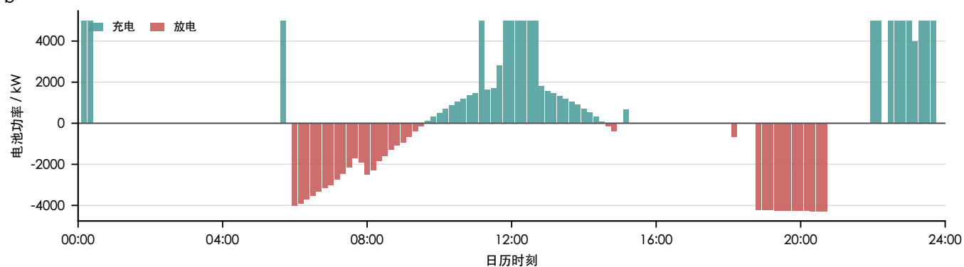
充放电动作 (充电为正, 放电为负)
