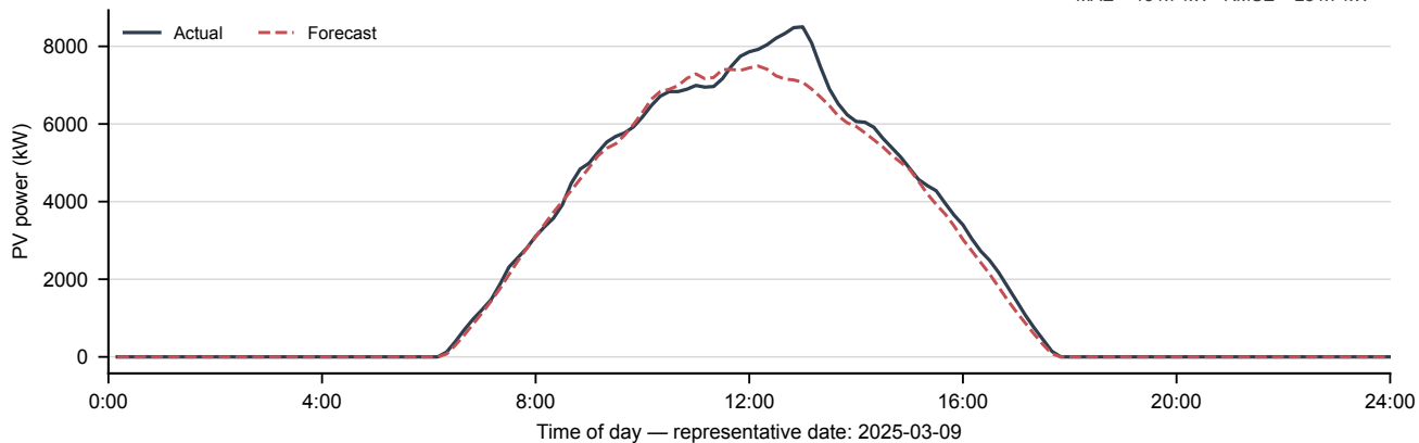
Actual and forecast PV
