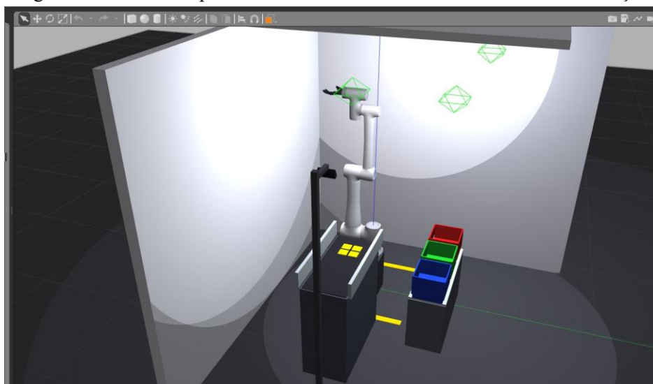
Figura 6 – Detalhe da pick station da esteira e das três caixas de classificação
