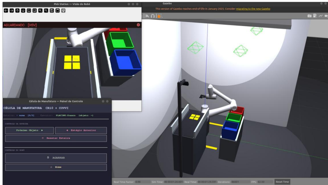
Figura 9 – Conjunto braço-mão em posição de aproximação à pick station no Gazebo
