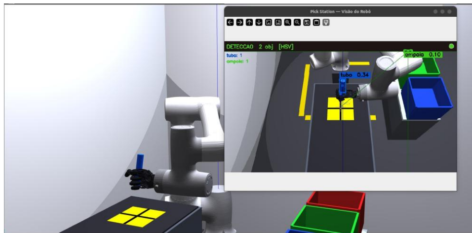
Figura 11 – Execução do claw grip sobre o tubo de ensaio (Box 2, caixa verde)
