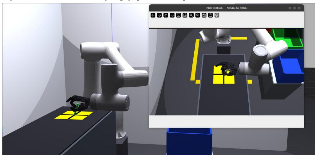
Figura 12 – Execução do fingertip grip sobre a ampola farmacêutica (Box 3, caixa azul)
