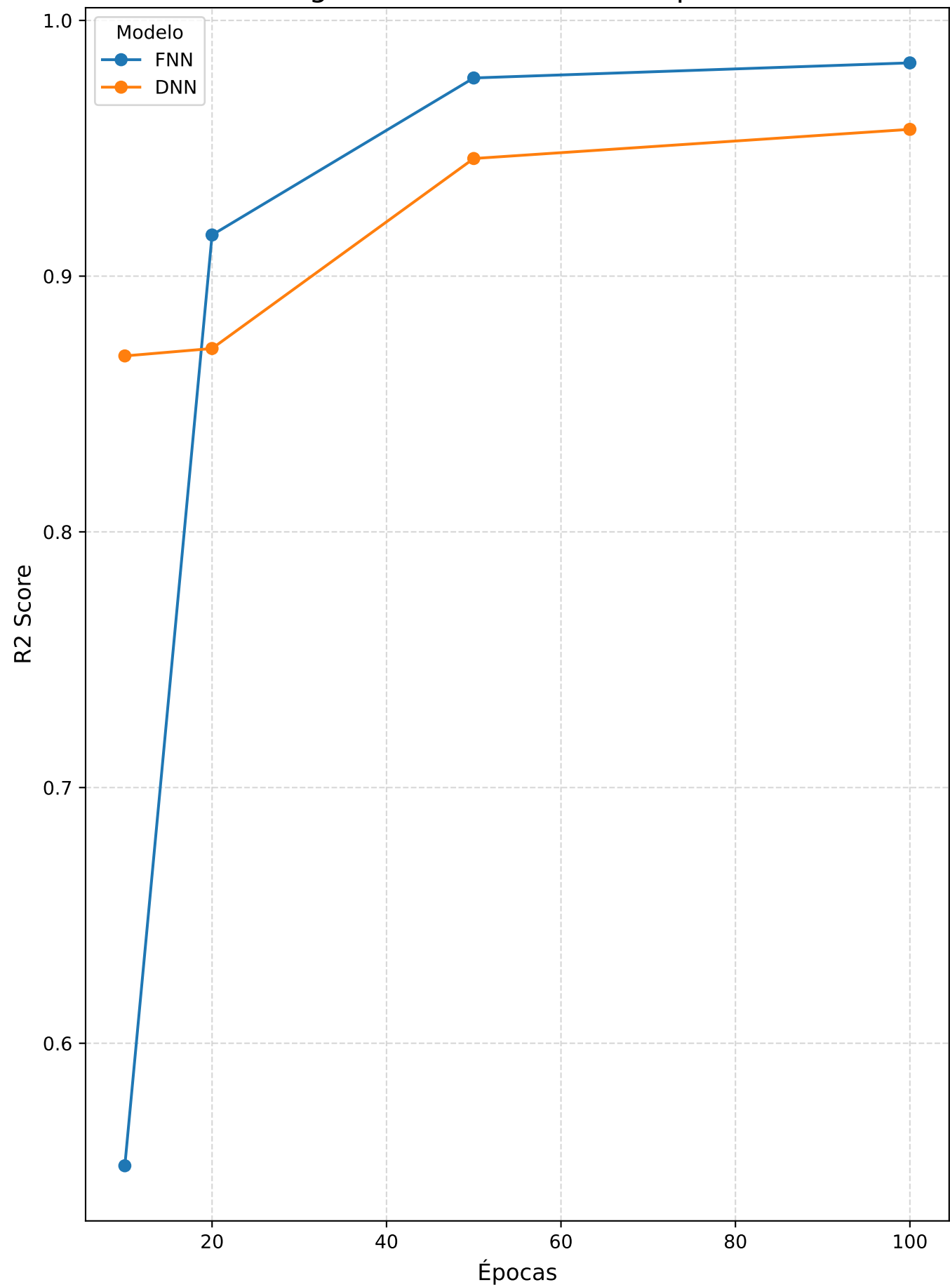
Regression • R2 Score vs Épocas
