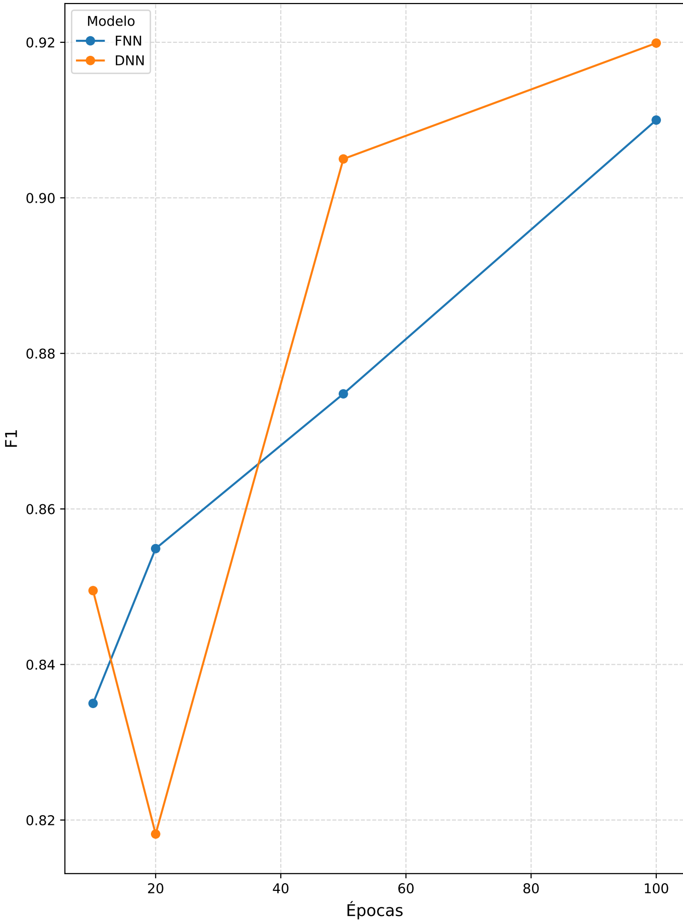
Classification • F1 vs Épocas
