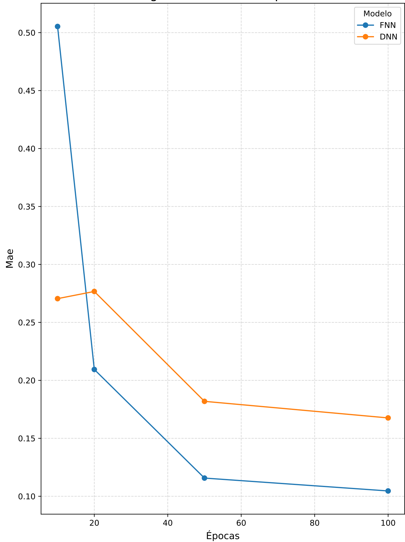
Regression • Mae vs Épocas
