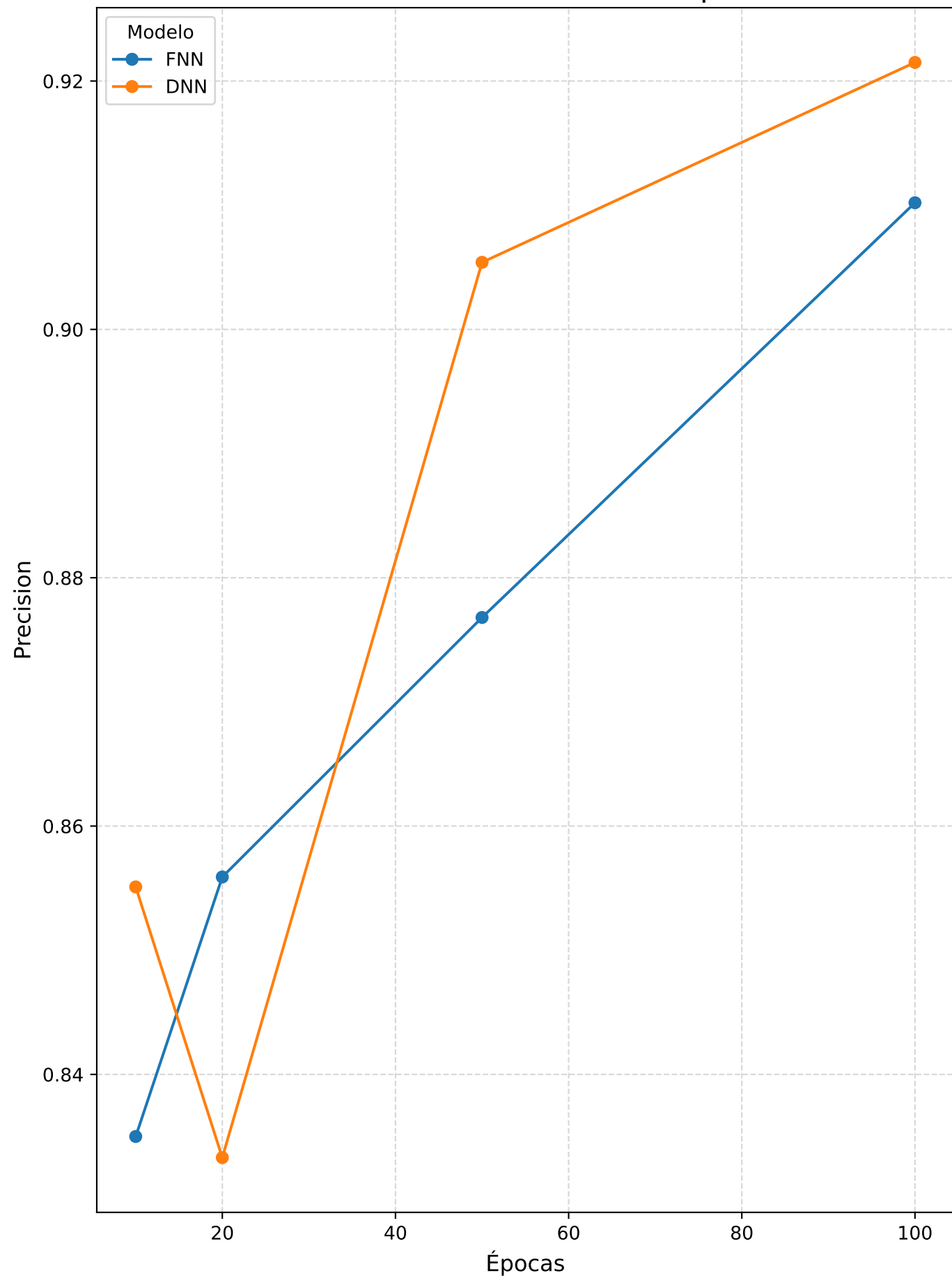
Classification • Precision vs Épocas
