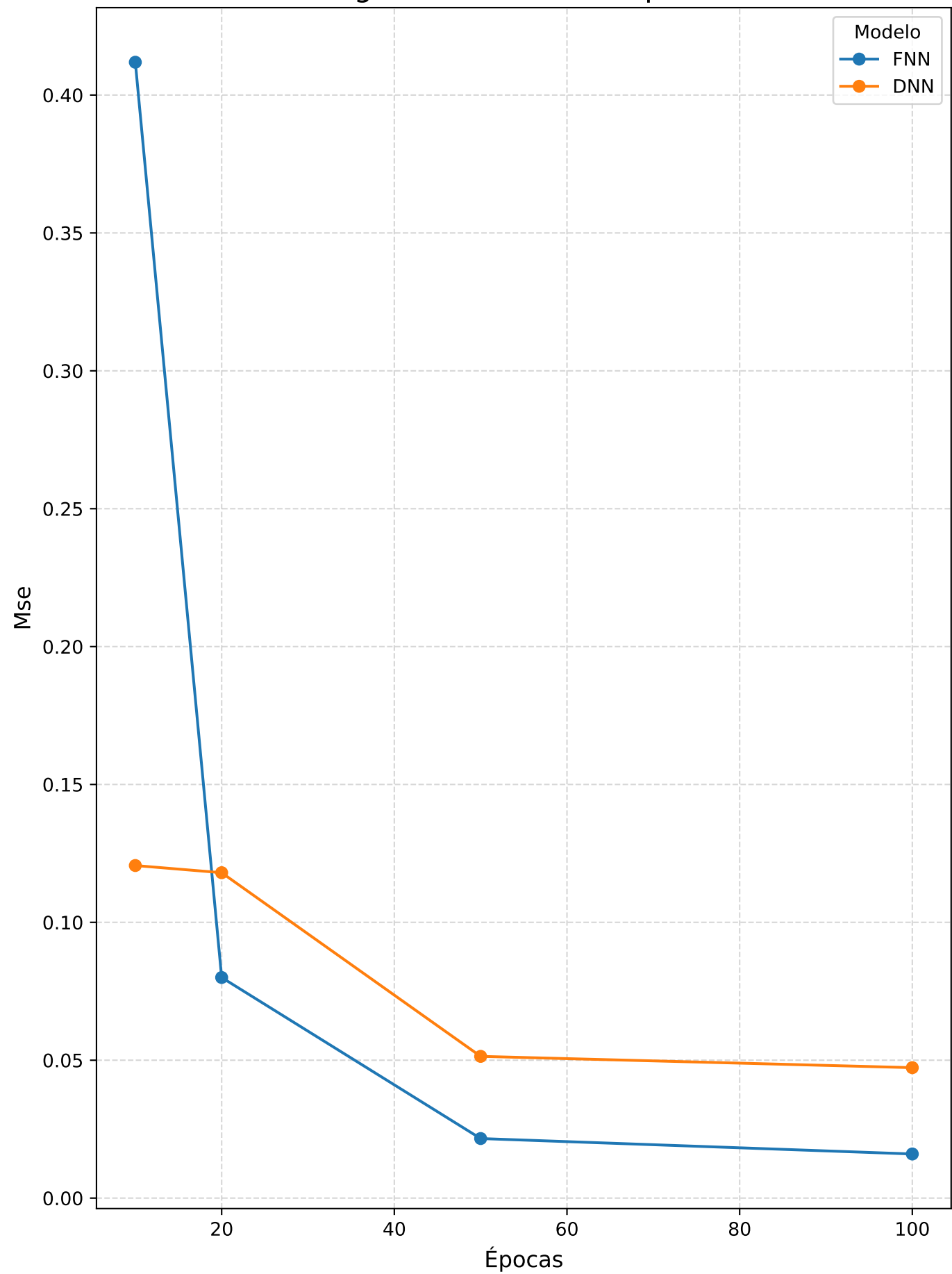
Regression • Mse vs Épocas
