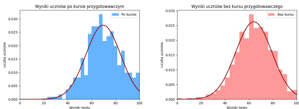
Rysunek 2: Histogramy (opisane powyżej) z nałożoną gęstością rozkładu normalnego (czerwona linia).
