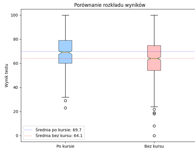
Rysunek 3: Wykresy pudełkowe z zaznaczonymi wartościami odstającymi oraz średniami.
