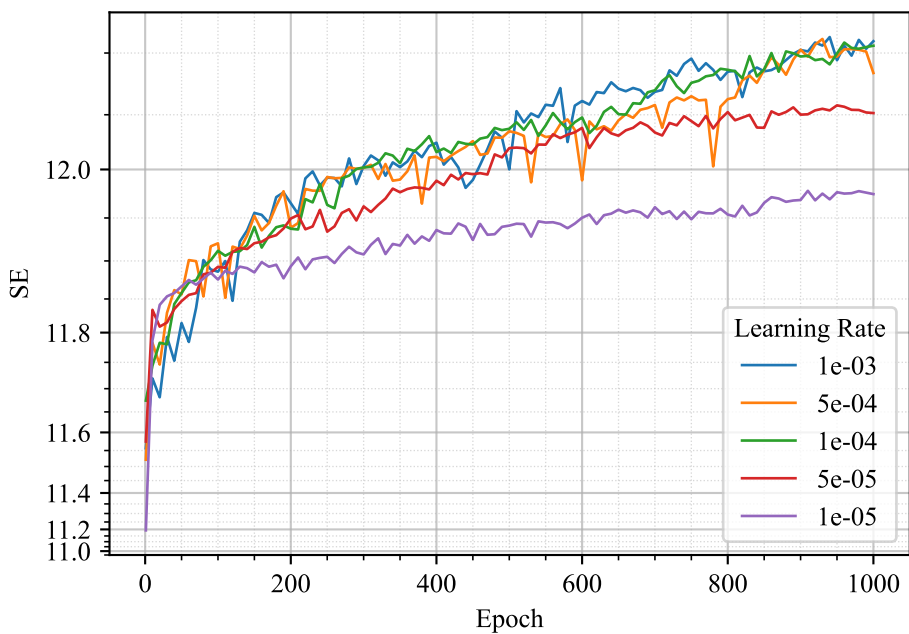
Validation SE
