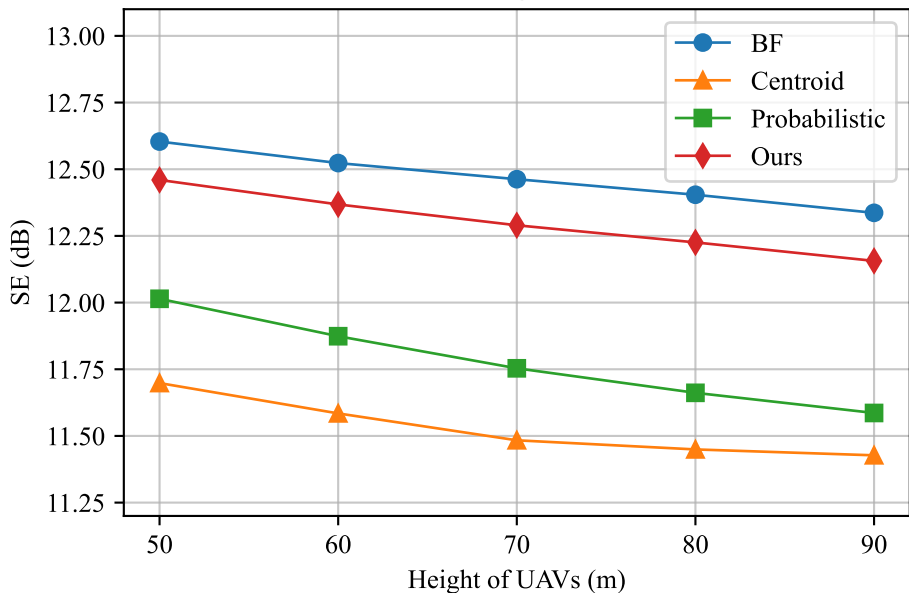
UAV Height vs SE
