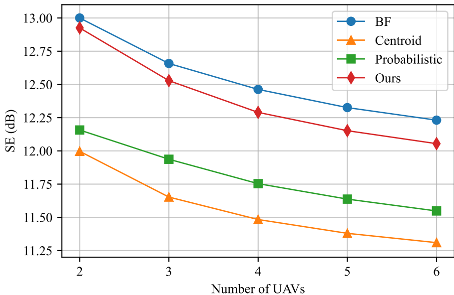
UAV Number vs SE
