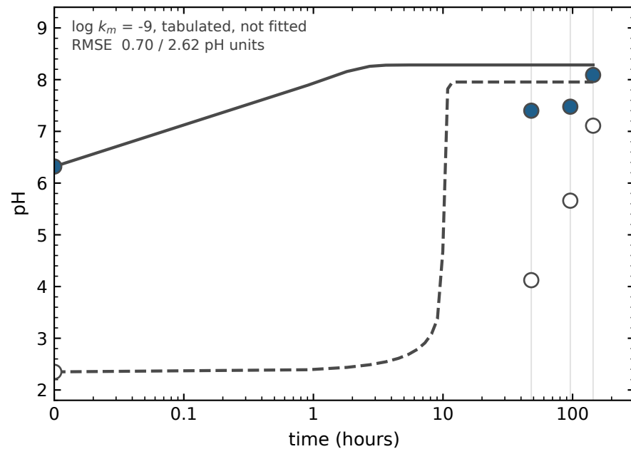
(D) pH
