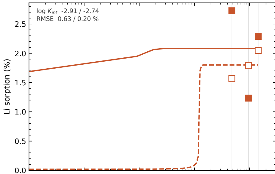
(B) pH
