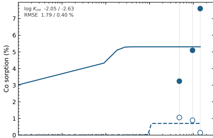
(D) pH
