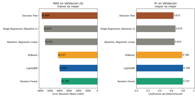
Figura 1. Comparación de MAE y R² en validación para los seis modelos evaluados.
