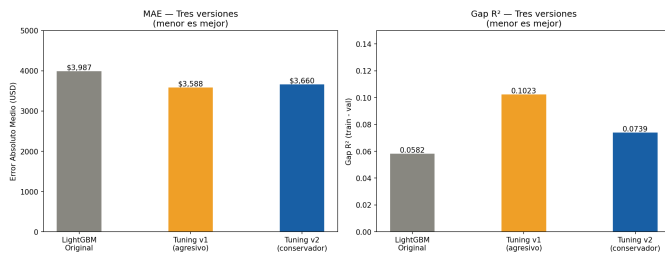
Figura 2. MAE y Gap R² para las tres versiones de LightGBM. Tuning v2 logra el mejor balance entre precisión y generalización.
