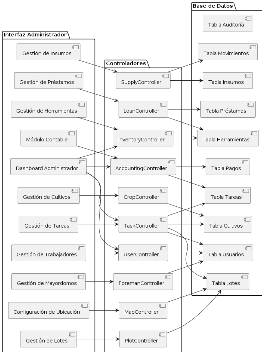
Diagrama de Componentes - Administrador AGROSAC
