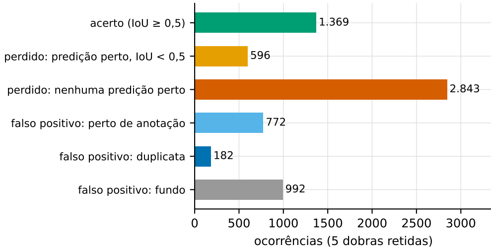
Config. 2: 4.808 anotações, 3.315 predições
