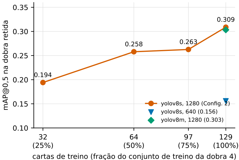
Curva de aprendizado, dobra 4
