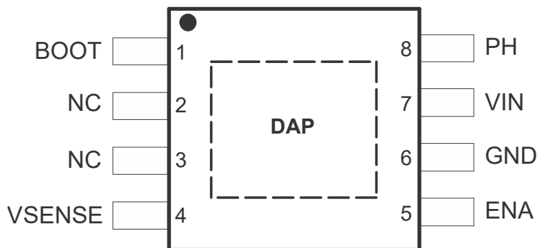
图 4-1. DDA 封装 8 引脚 HSOIC (带散热焊盘) (顶视图)
