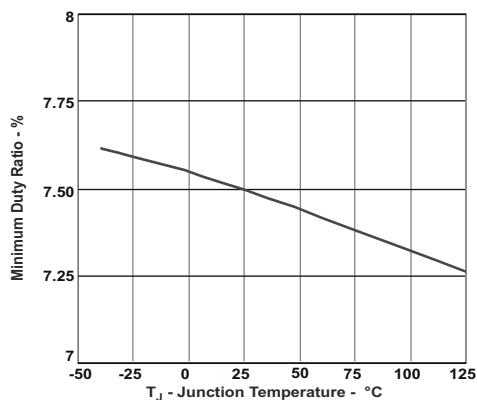
图 5-8. 最小可控占空比与结温间的关系
