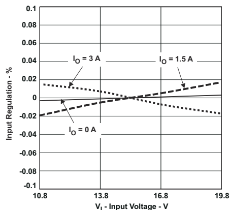
图 7-4. 输入调节百分比与输入电压的关系
