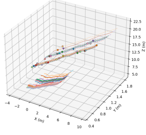
baseline
