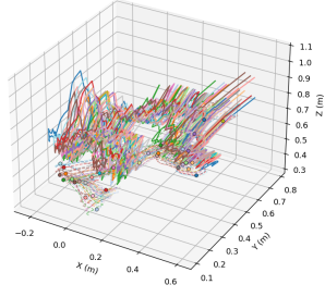
baseline
