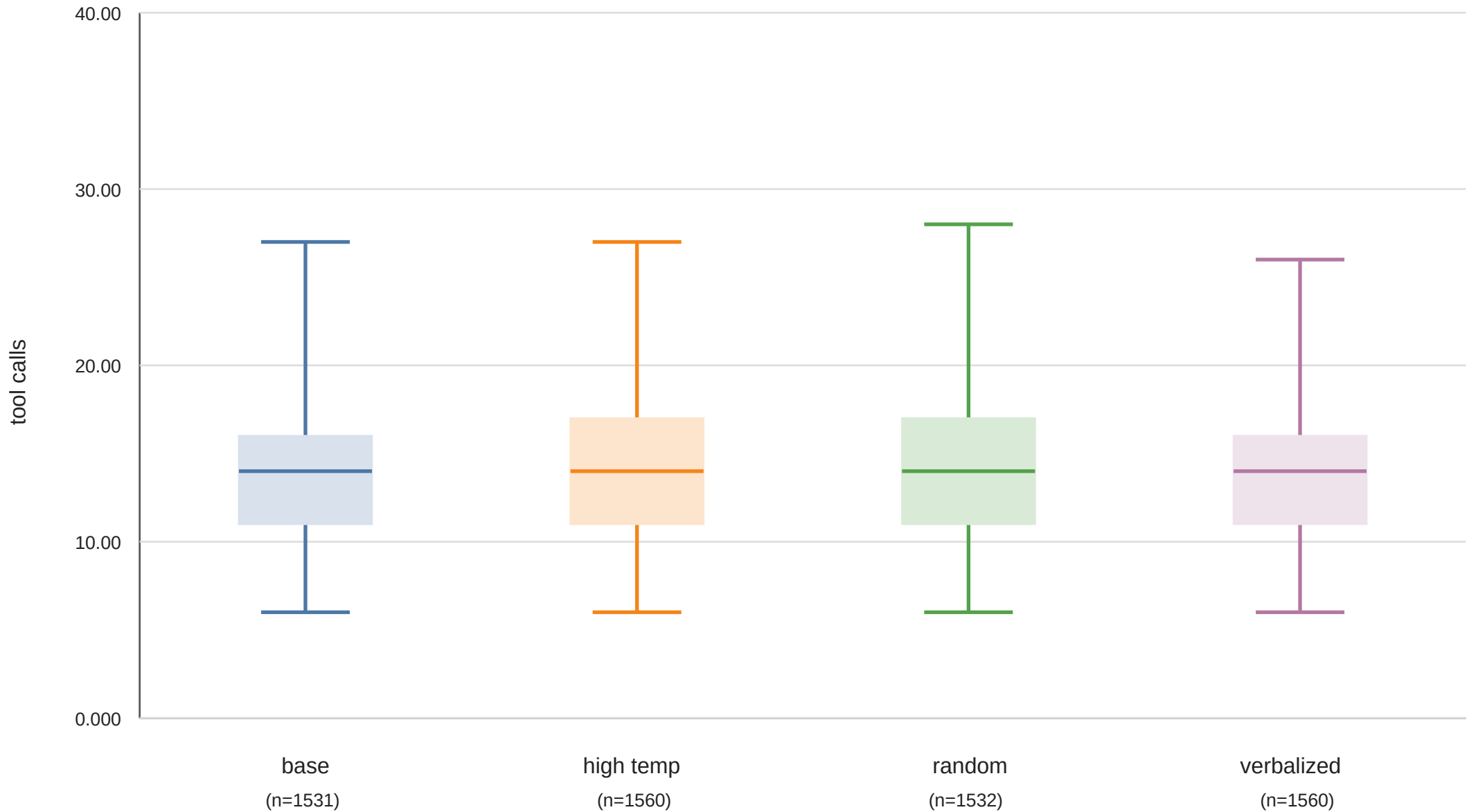
Tool calls per trajectory
