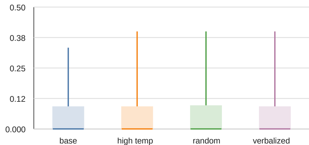
place_on_object
