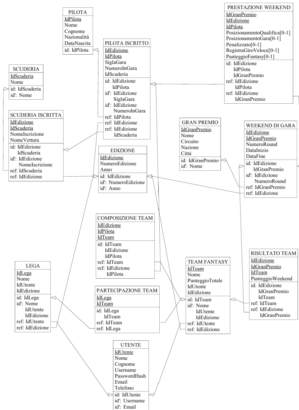
Figura 3.7: Schema logico relazionale finale
