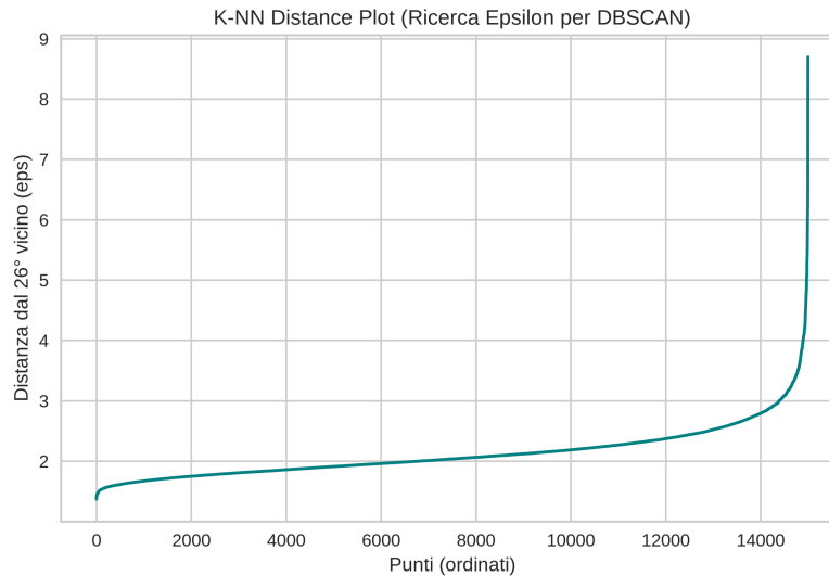
Figura 4: Grafico delle distanze K-NN per la determinazione dell’epsilon ottimale del DBSCAN. Il punto di ginocchio è stato individuato nella regione \varepsilon \approx 2.6 .
