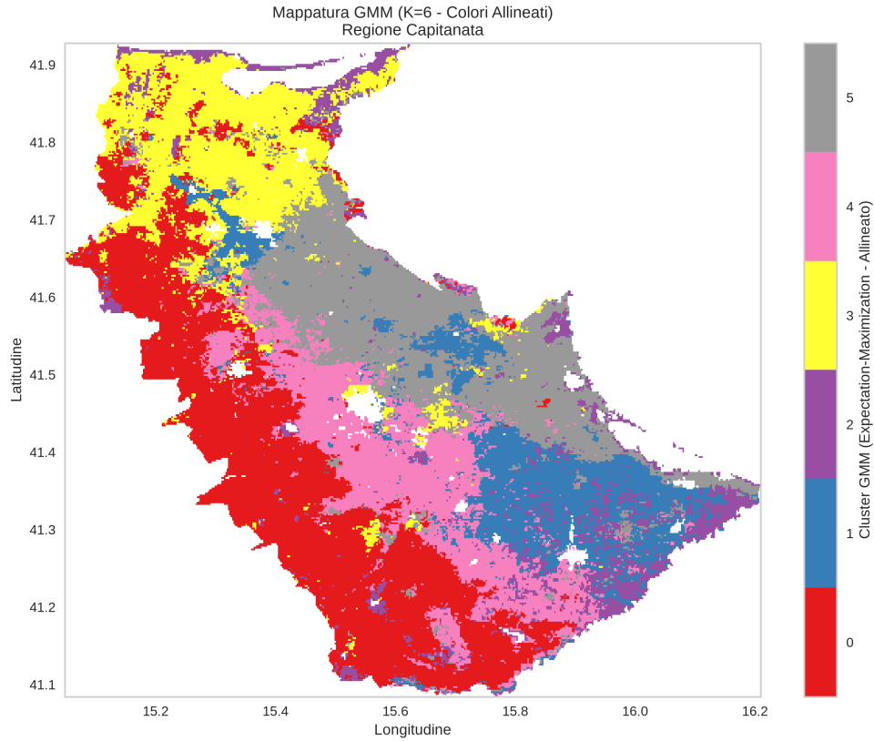
Figura 13: Mappatura spaziale dei cluster GMM con K=6 . L'assegnazione è basata sulla componente gaussiana con probabilità a posteriori massima ( hard assignment ). Le etichette sono allineate al K -Means per confronto diretto.
