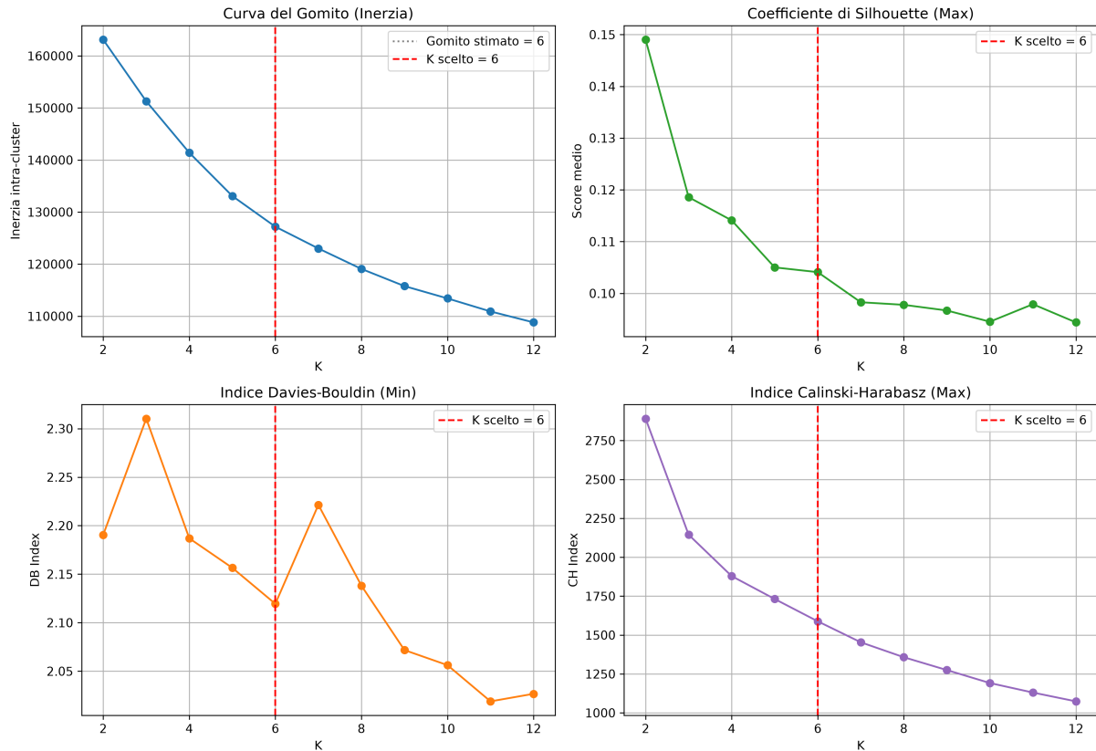
Figura 5: Le quattro metriche per la selezione del K ottimale: Curva del Gomito (Inerzia), Coefficiente di Silhouette, Indice di Davies-Bouldin e Indice di Calinski-Harabasz. La linea tratteggiata rossa indica K = 6 .
