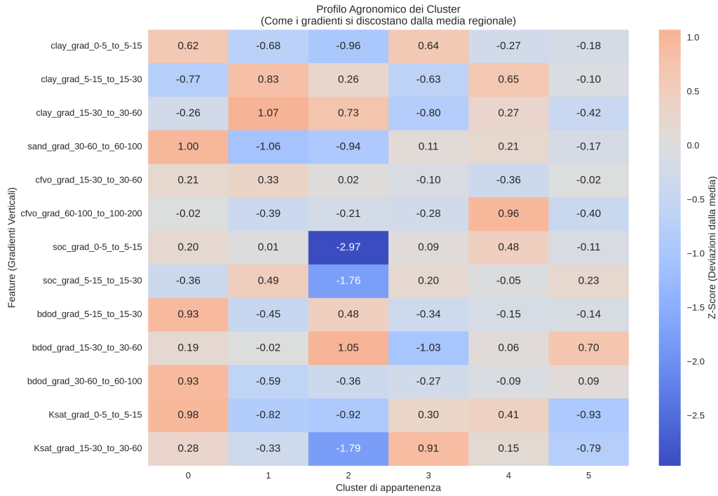
Figura 11: Profilo agronomico dei 6 cluster basato sugli Z-score dei centroidi. Valori positivi (rossi) indicano gradienti superiori alla media regionale; valori negativi (blu) indicano gradienti inferiori.
