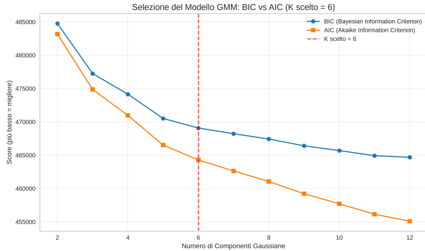
Figura 12: Curve BIC e AIC per il GMM al variare del numero di componenti. La linea tratteggiata rossa indica K = 6 .
