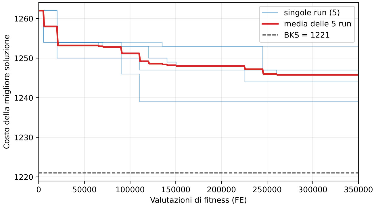
Convergenza su B-n78-k10
