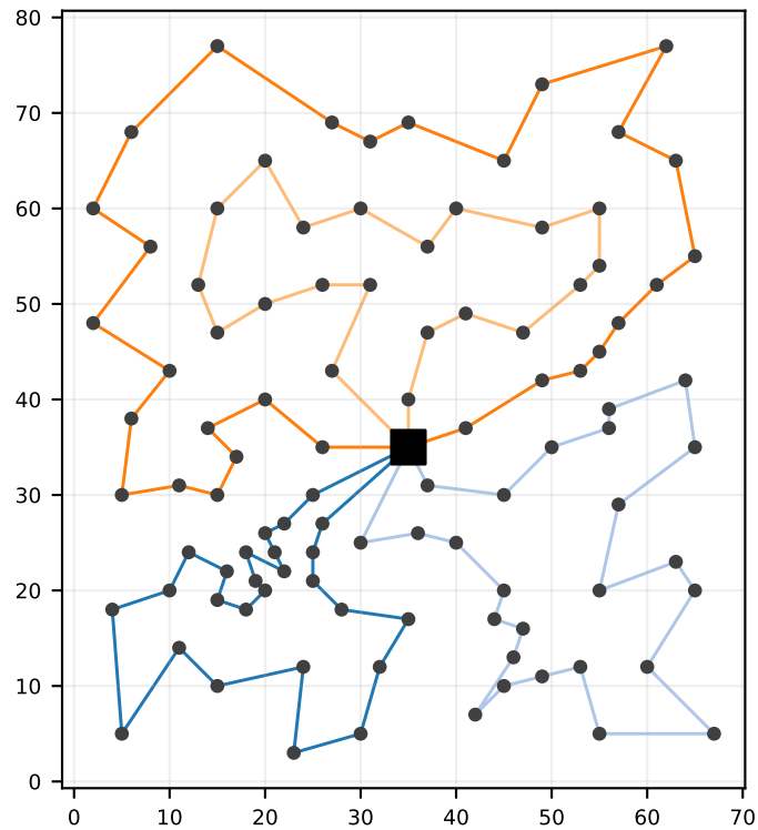
Soluzione ottima (CVRPLIB) — costo 681 4 rotte
