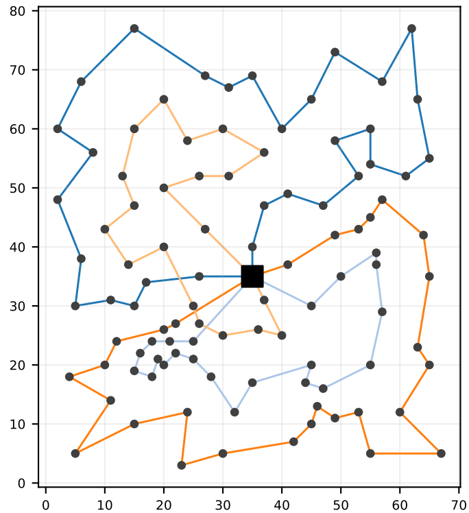
Soluzione trovata — costo 719 (gap 5.58%) 4 rotte, seed 0
