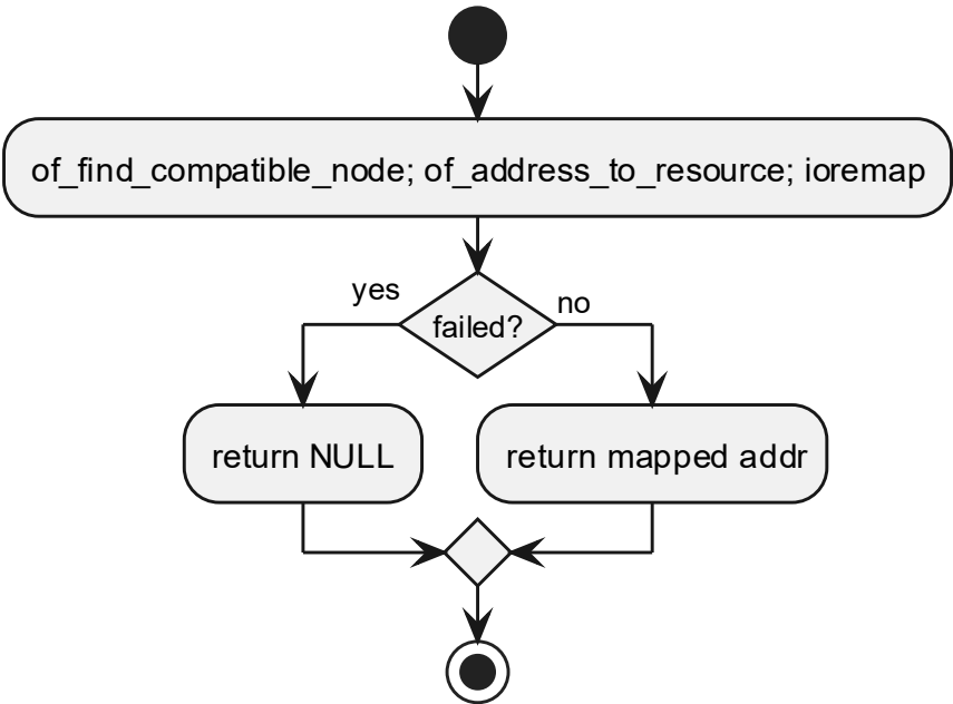
6.7.13 ipcsOsMapIntc processing flow
