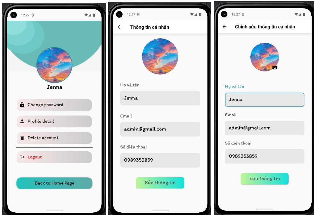
Hình 3: Giao diện xem, sửa thông tin cá nhân
