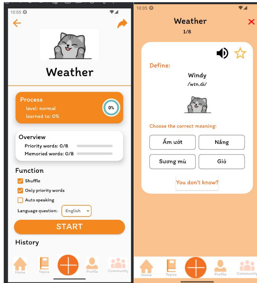
Hình 12: Chỉnh sửa thông số trước khi tạo bài trắc nghiệm và giao diện trắc nghiệm
