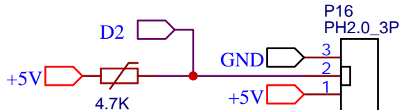
Connessione sensore di Temperatura
