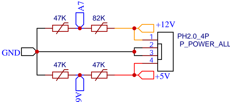
Connessione Alimentazione +12V +5V + Voltmetro Analogico della +12v +5V
