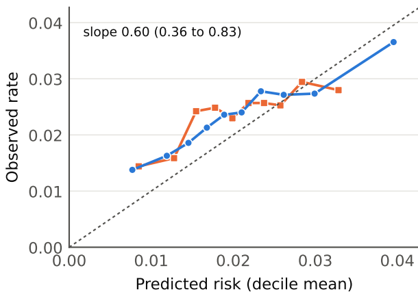
C Calibration, shoulder IL
