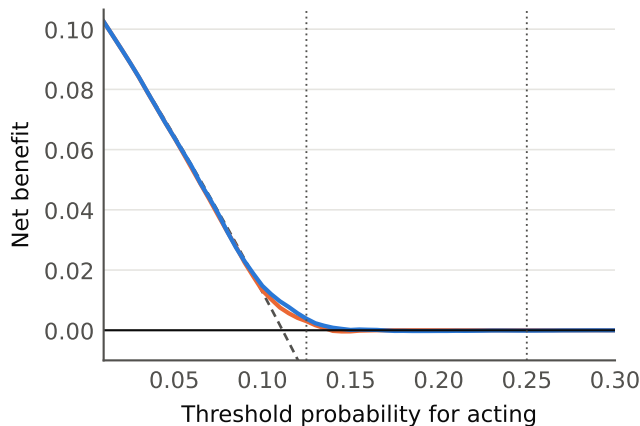
B Decision curve, any IL
