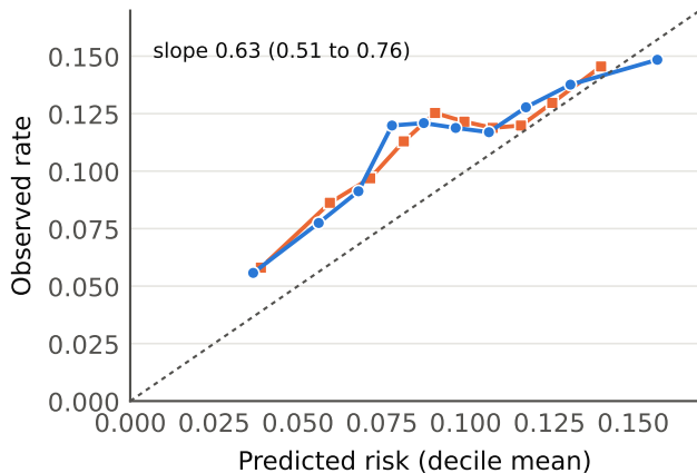
A Calibration, any IL
