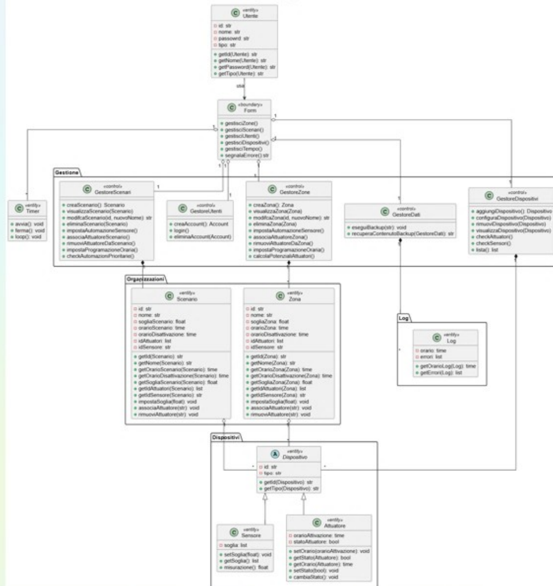
Smart Home diagramma di progettazione delle classi
