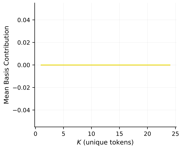
MLP Hidden
