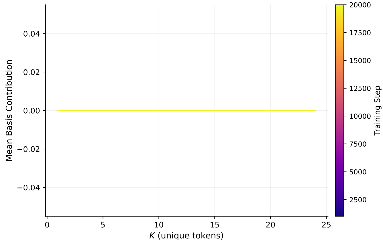
MLP Hidden
