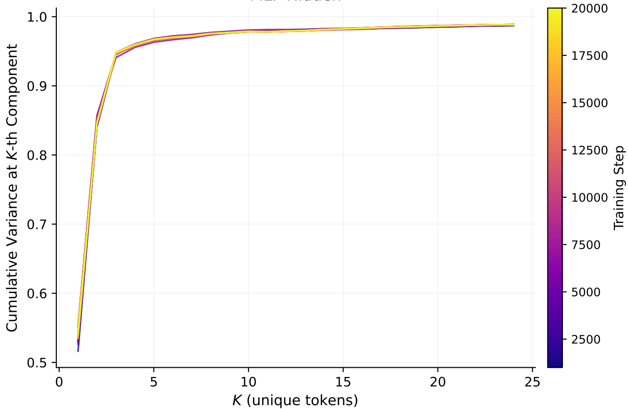
MLP Hidden
