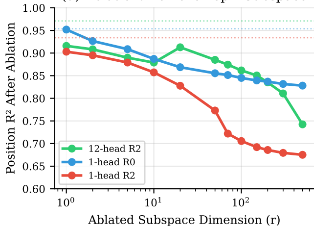
(d) Ablation: Remove Top-r Subspace
