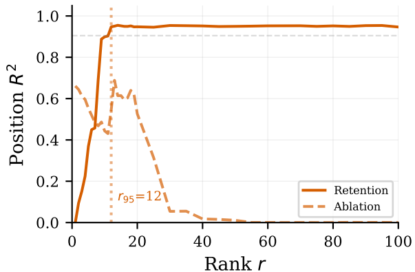
R2
