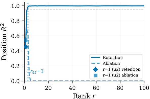
R0
