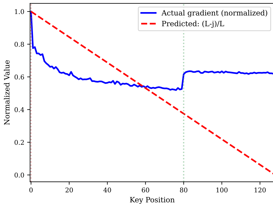
Actual vs Predicted Gradient Pattern
